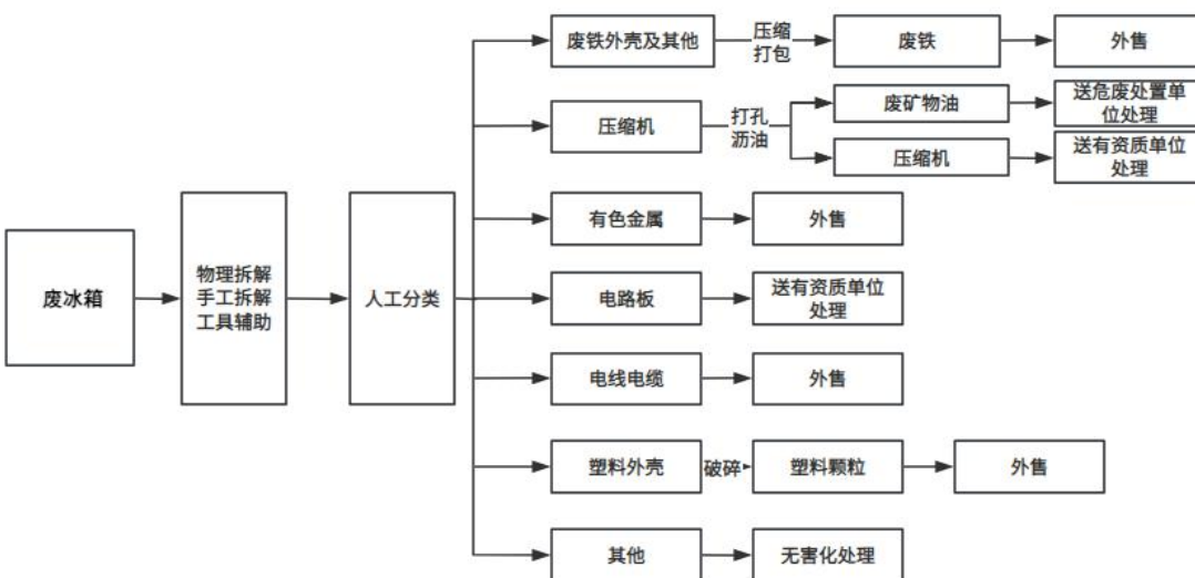
图 2.13-4 现有项目废冰箱拆解工艺流程图
