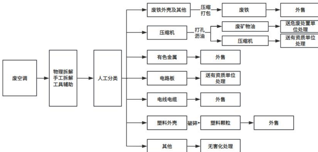
图 2.13-3 现有项目废空调拆解工艺流程图
