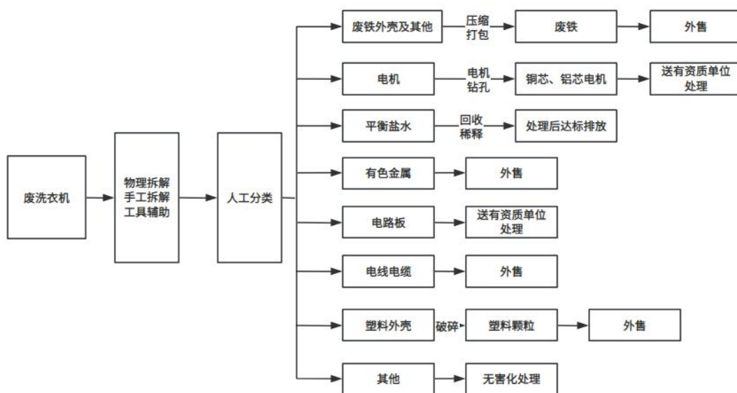
图 2.13-2 现有项目废洗衣机拆解工艺流程图
