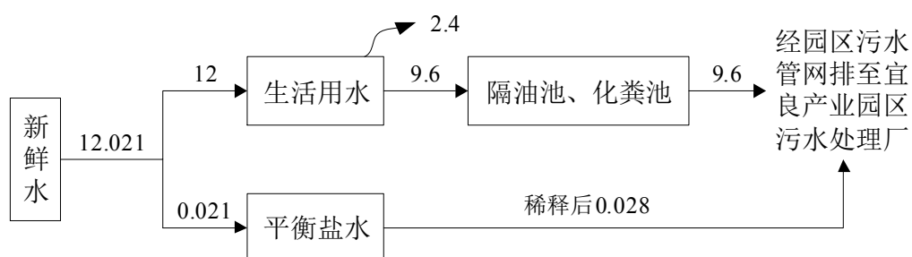
图 4.2.2-2 项目雨天水平衡图 (单位: \text{m}^3/\text{d} )
