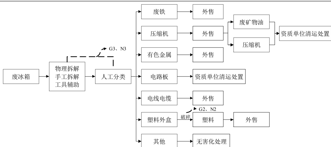
图 2.11-3 冰箱拆解线工艺流程及产污节点示意图
