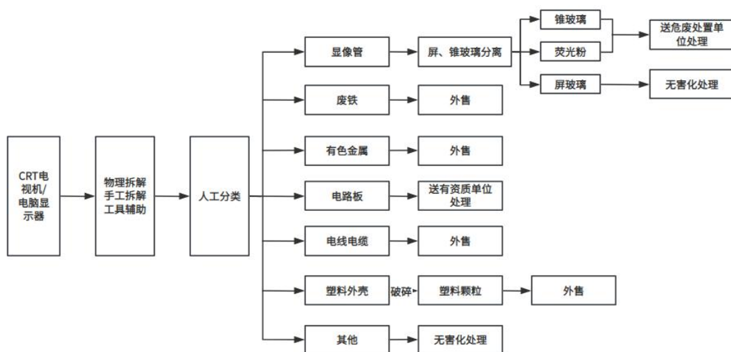
图 2.13-1 现有项目电视/电脑显示器拆解工艺流程图
