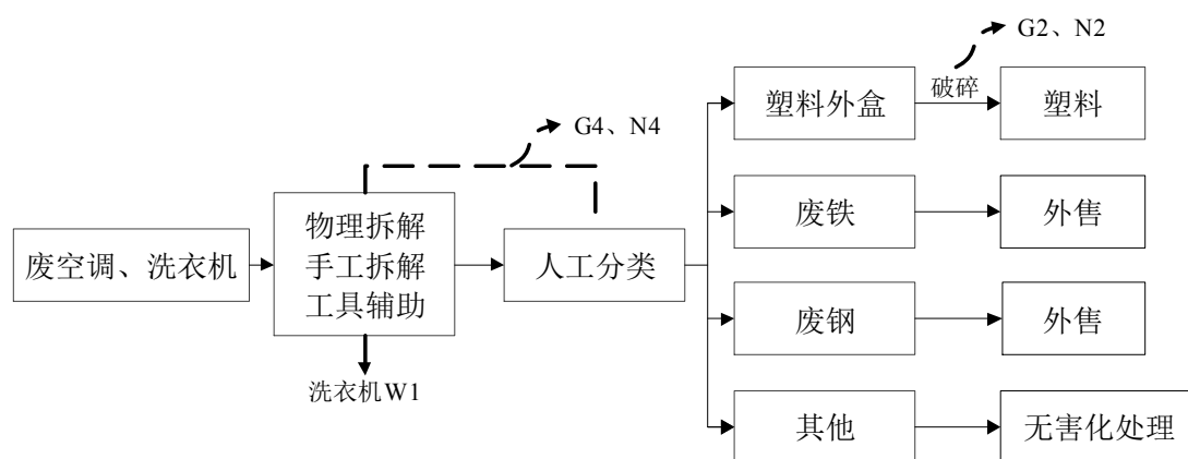
图 2.11-2 洗衣机、空调综合拆解线工艺流程及产污节点示意图
