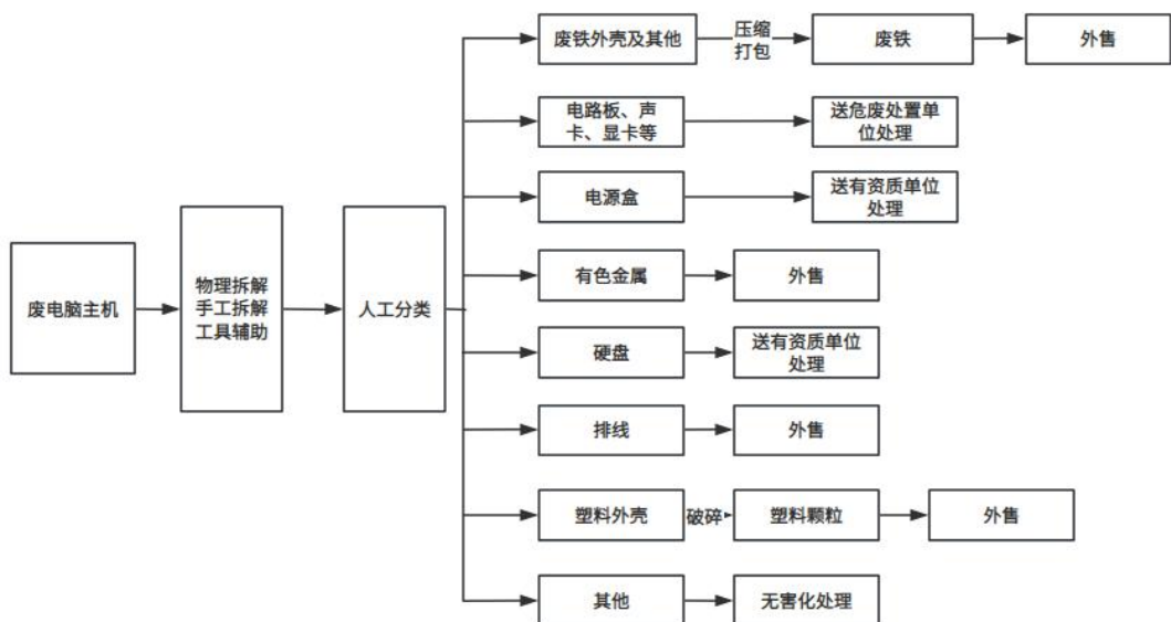
图 2.13-5 现有项目废电脑主机拆解工艺流程图
