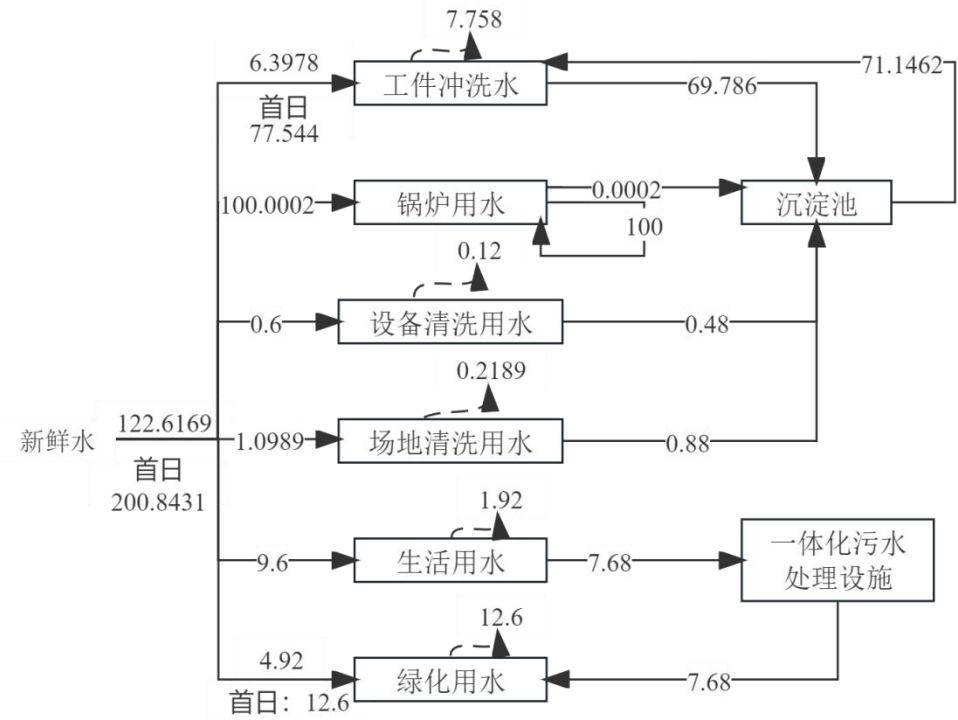
图 2-1 晴天水平衡图 m 3 /d
