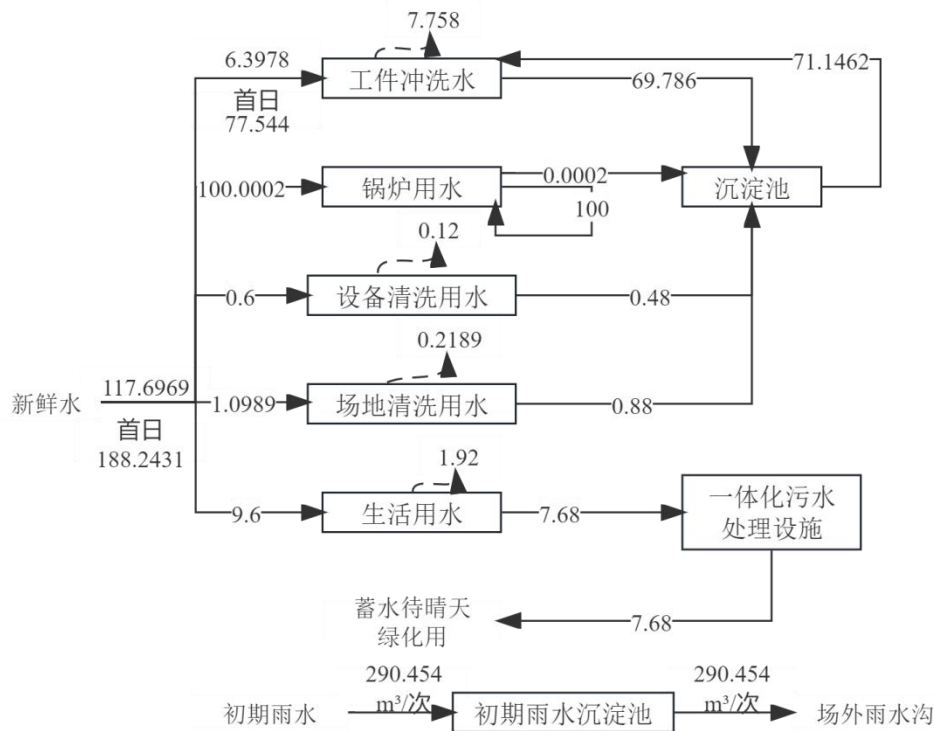
图 2-2 雨天水平衡图
