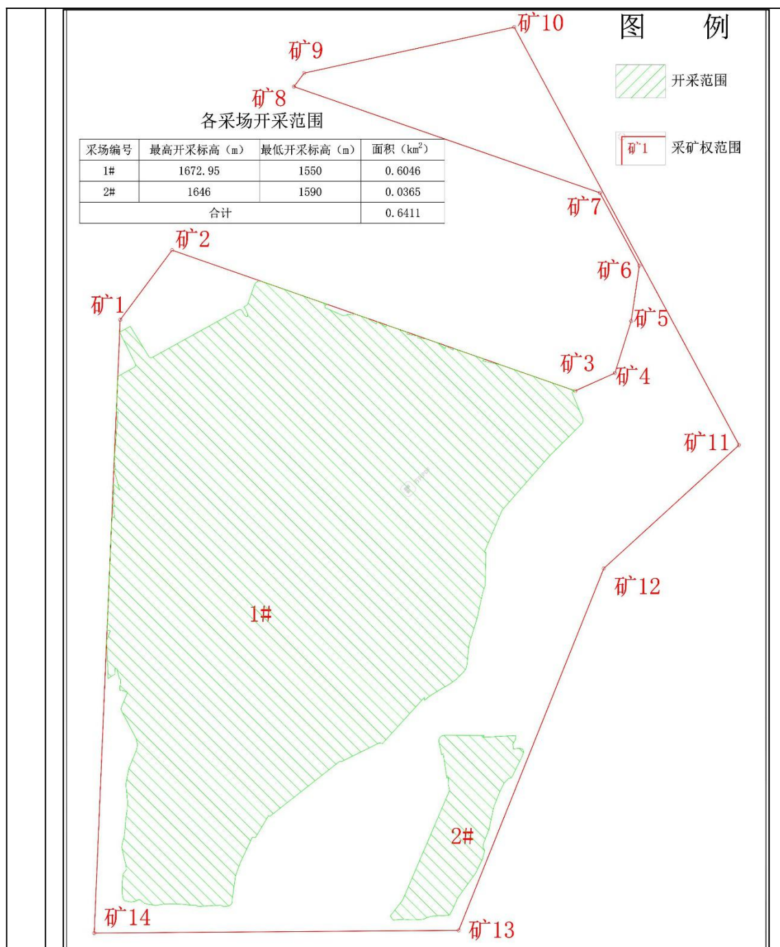
图 2-1 开采境界范围图
