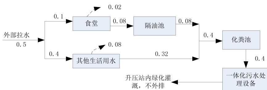
图 4-5 项目运营期水平衡图
