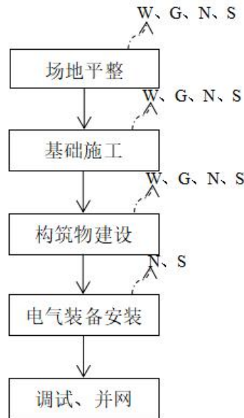
图 2-6 升压站施工工艺流程及产污节点示意图
