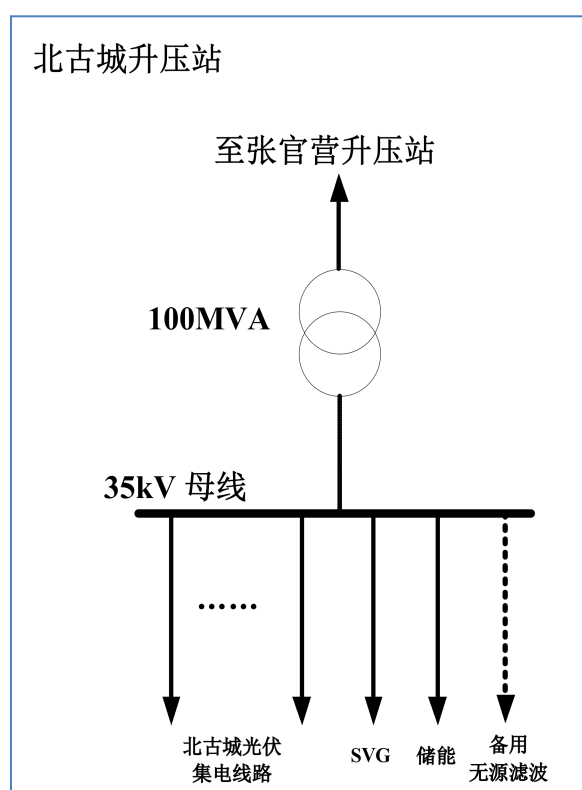
图 2-2 北古城升压站 110kV 出线间隔布置图
