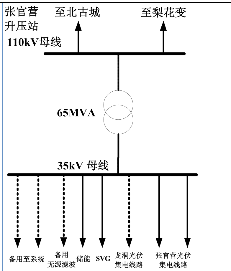
图2-3 张官营光伏电站110kV升压站本期110kV出线间隔示意图
