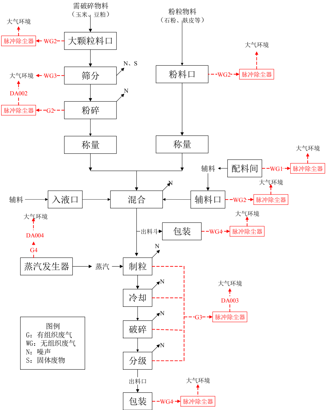
图 2.2-3 浓缩饲料生产线工艺流程及产排污节点图
