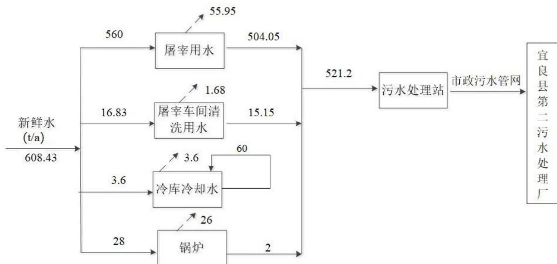
图 5.2.4 本扩建项目水平衡图
