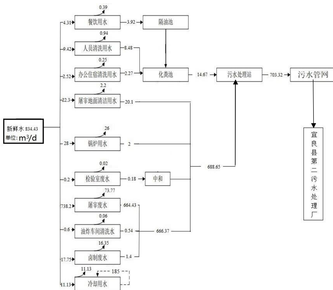
图 5.2.6 扩建后全厂水平衡图
