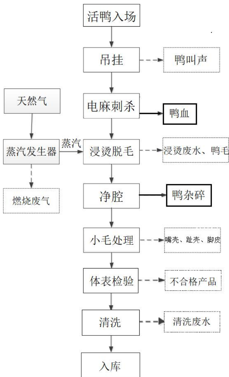
图 5.2.1 白条鸭生产工艺流程图
