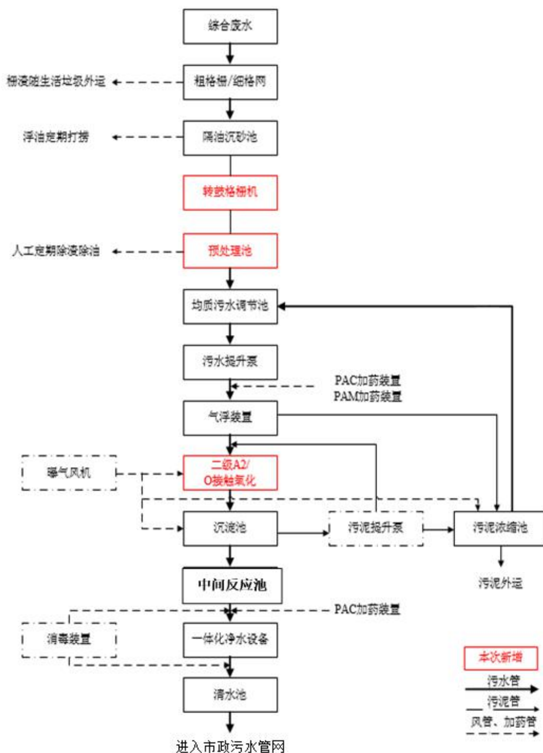
图 5.2.2 污水处理工艺流程图
