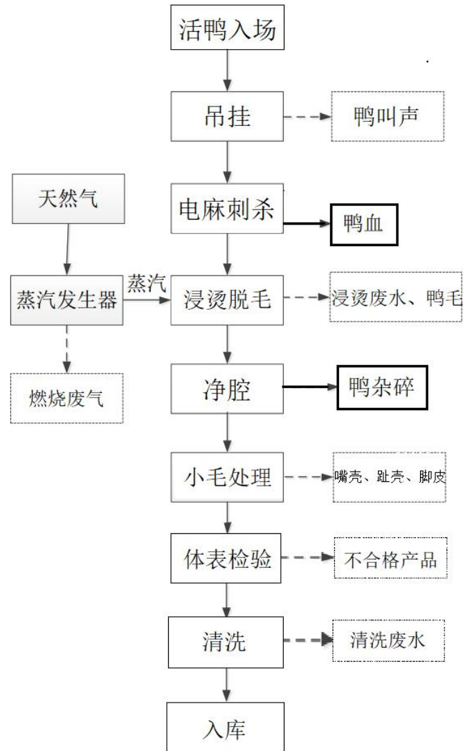
图 3.3.1 白条鸭生产工艺流程图
