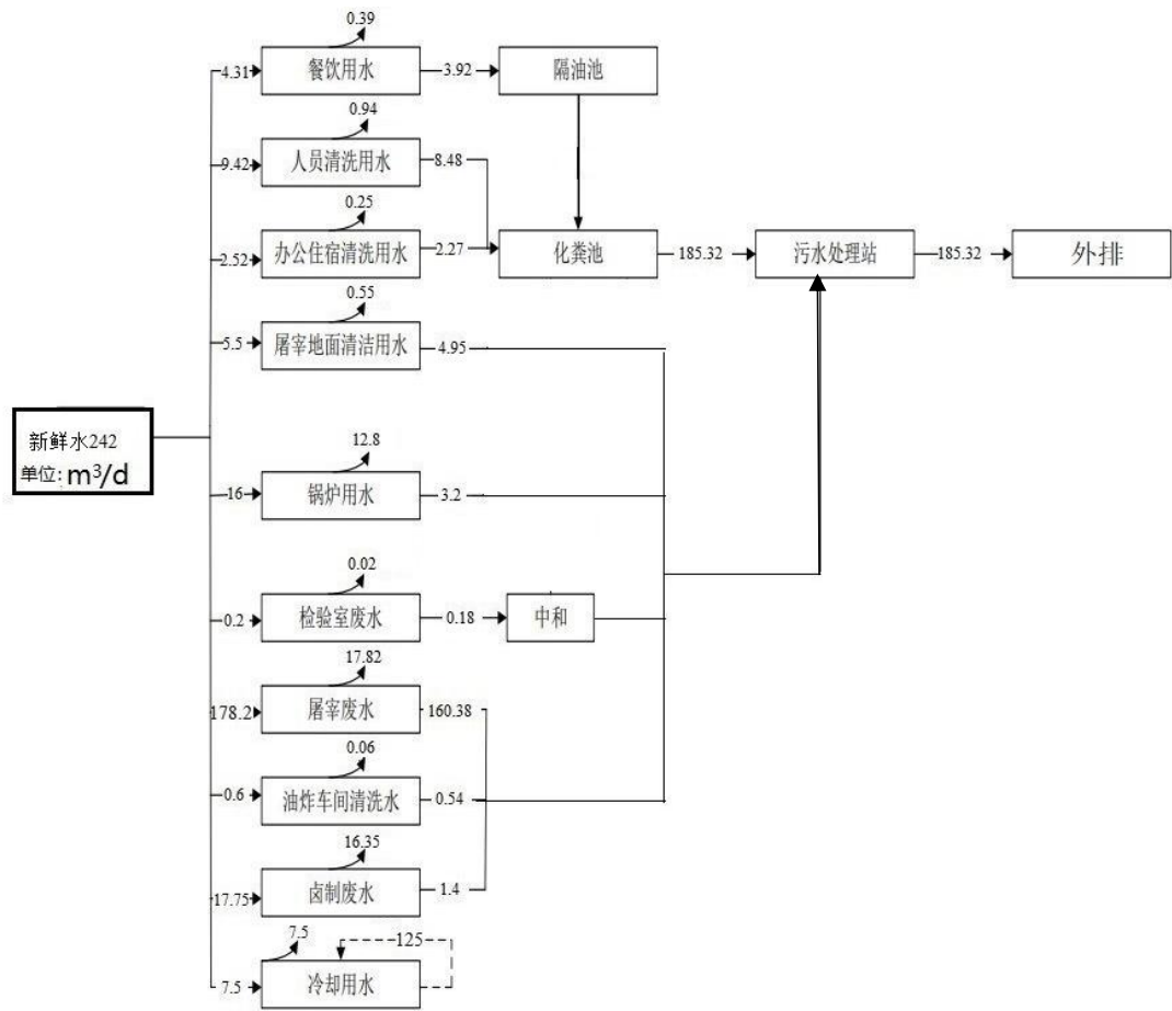
图 3.4.2 原项目水平衡图
