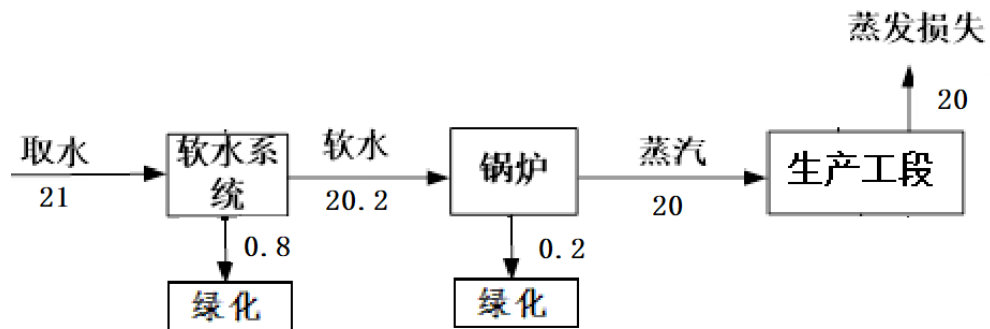
图 2-2 远期天然气锅炉水平衡图(m³/d)
