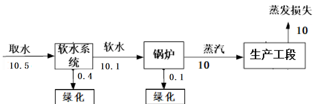
图 2-3 现有项目锅炉房水平衡图(m 3 /d)
