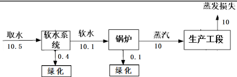
图 2-1 近期天然气锅炉水平衡图(m³/d)
